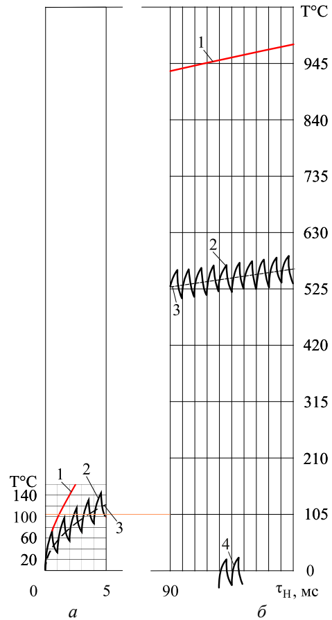
Рис. 3. Температура ( T °C) прерывистого шлифования при N = 35 на интервале времени переходного процесса (а) и установившаяся температура (б)
