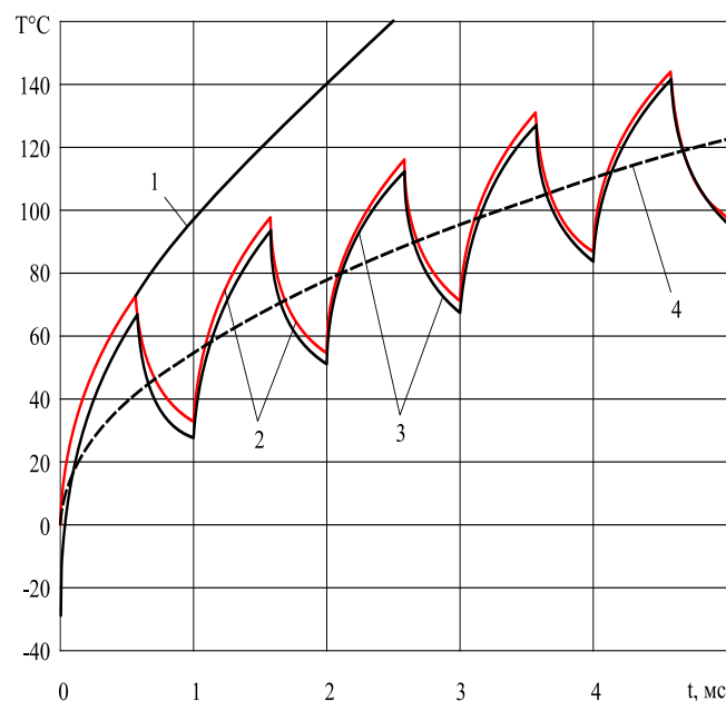
Рис. 2. Температура шлифования в начале нагрева на участке переходного процесса:
