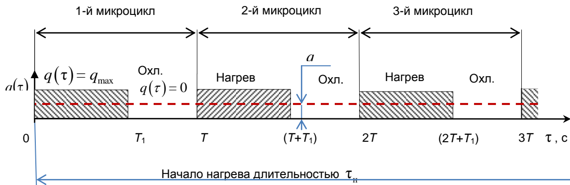
Рис. 1. Периодический тепловой поток с плотностью q(\tau) :
